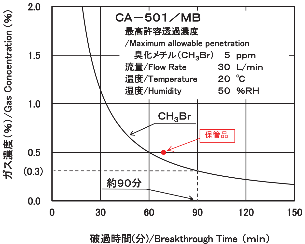
図 CA-501/MB (臭化メチル用) の臭化メチルに対する破過曲線
