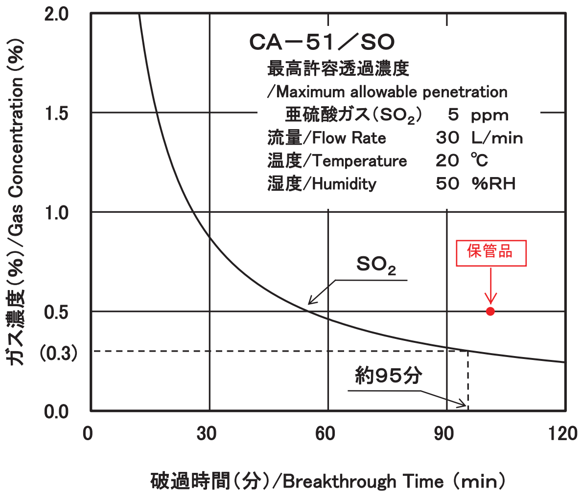
図 CA-51/SO (亜硫酸ガス用) の 亜硫酸ガスに対する破過曲線
