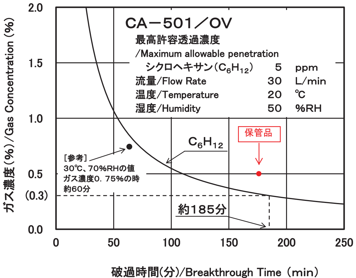
図 CA-501/OV (有機ガス用) のシクロヘキサンに対する破過曲線
