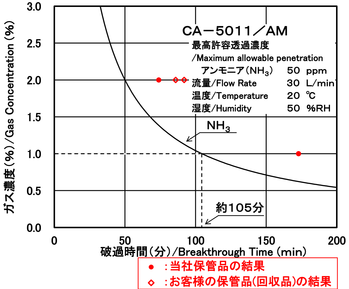
図 CA-5011/AM (アンモニア用) のアンモニアに対する破過曲線
