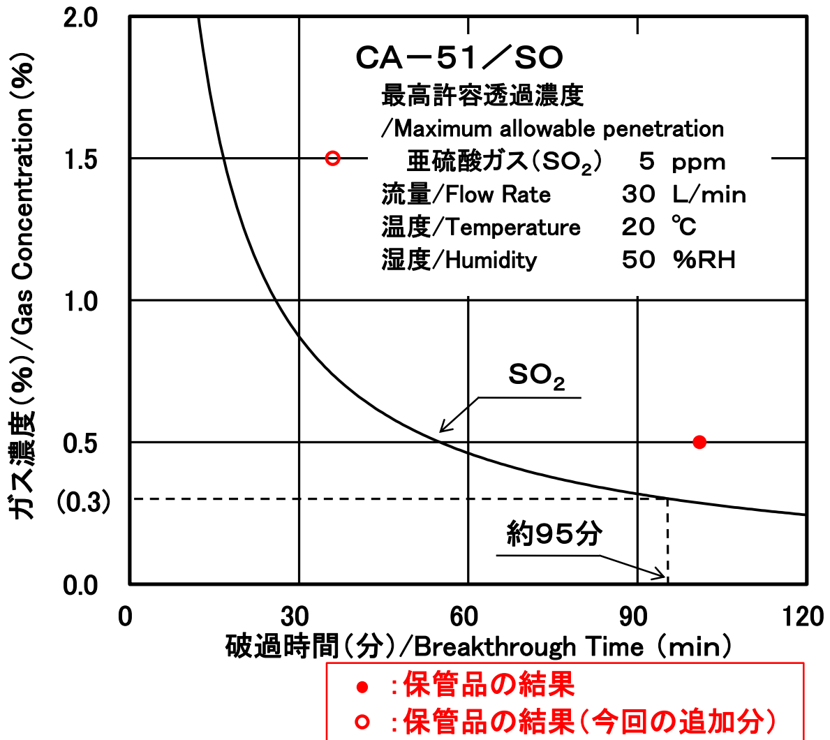
図 CA-51/SO (亜硫酸ガス用) の 亜硫酸ガスに対する破過曲線
