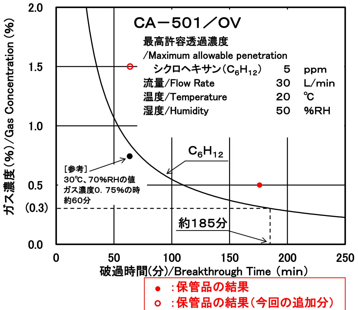
図 CA-501/OV (有機ガス用) のシクロヘキサンに対する破過曲線
